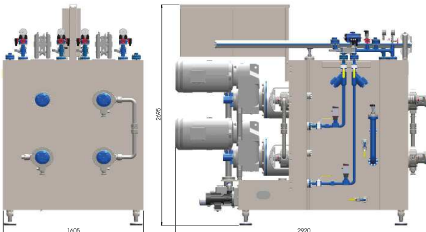
Polaron A+B+C+D CO2, cascade system
