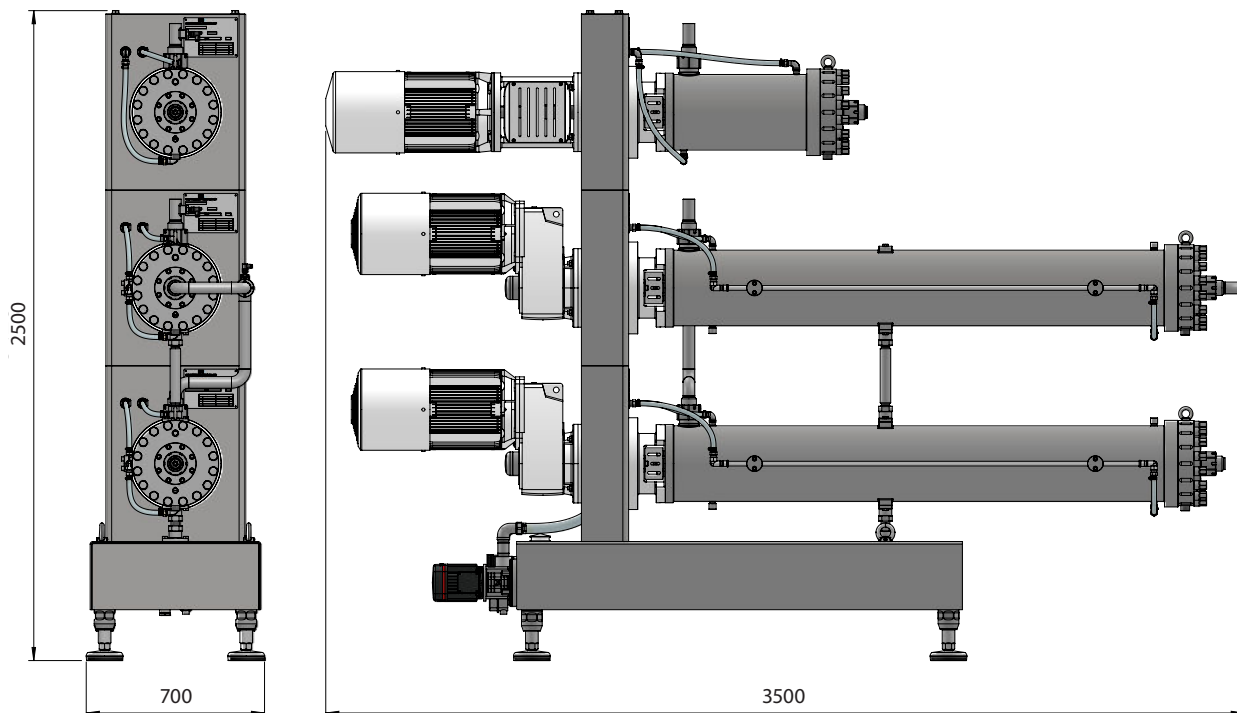
POLARON PIN ROTOR MACHINE 2X80 L. AND POLARON PLASTICATOR 25 L.
